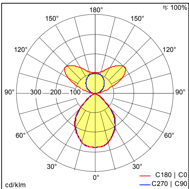
D43607AA_CLEVO_ID_LED_12000-840_L3080_LDO_SR_SRG.Idt
