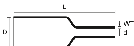
Gaine thermorétractable 4:1
