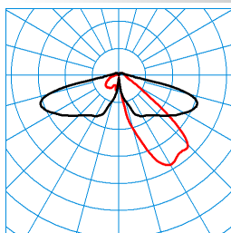
8841LS-Ü 360-AB2L/1000-730 2G2 ET (CLOANFANGSWERT) TX369394 ■ C0 - C180 ■ C90 - C270 DIN 5040: A20 UTE: 0,92 I + 0,08 T CEN Flux Code: 29 64 91 92 100 12 33 60 8
