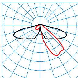
8841LS-Ü 360-AB2L/1000-730 2G2 ET (CLOENDWERT) TX369485 ■ C0 - C180 ■ C90 - C270 DIN 5040: A20 UTE: 0,92 I + 0,08 T CEN Flux Code: 29 64 91 92 100 12 33 60 8
