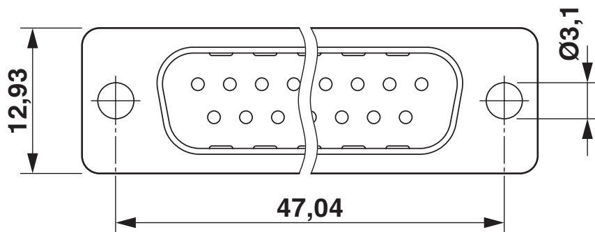
Dessin schématique
