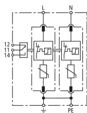
Schéma de principe du circuit DG M TN 275 FM
