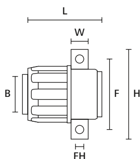
Raccord FlexiGuard, droit avec support
