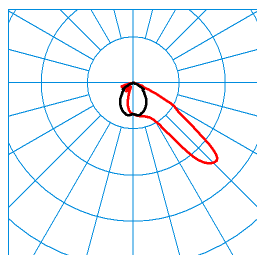
Jovie 50I-AM2L-LRA/6800-740 6G1 ET (CLO end value) TX300177 ■ C0 - C180 ■ C90 - C270 DIN 5040: A40 UTE: 1,00 F CEN Flux Code: 47 91 100 100 100
