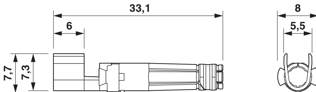
Dessin coté
