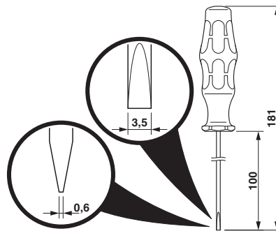
Dessin coté
