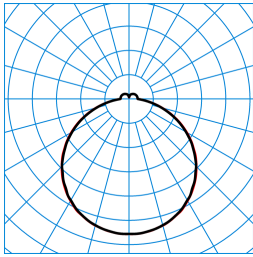
Olisq QWD2 DW 20-840 ET HFS IP54 IK TX77369
