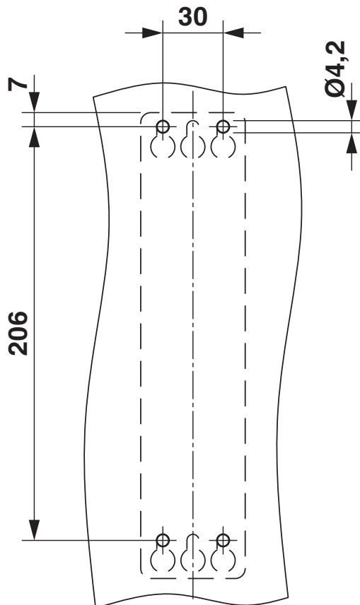
Gabarit perçage / géom. pastille soudage
