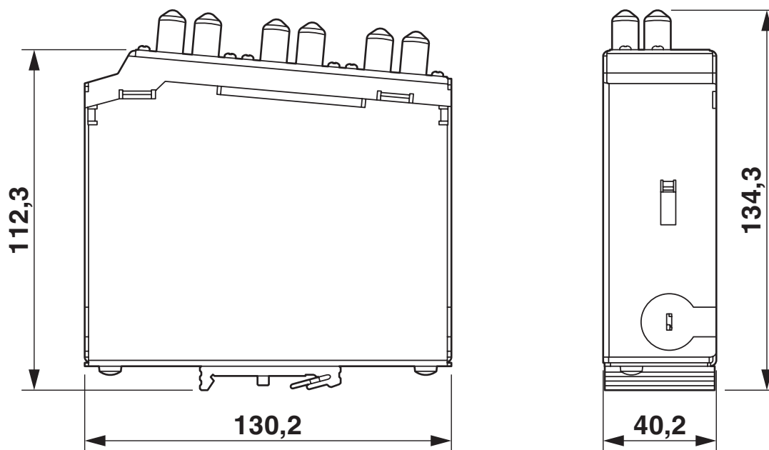
Dessin coté
