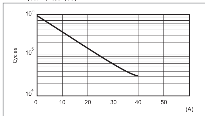
F 68-1 - Durée de vie électrique en fonction de la charge (AC1/AC7a) (68.24/25/54/55)
