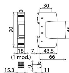
Dimensions DR M 2P 30 FM
