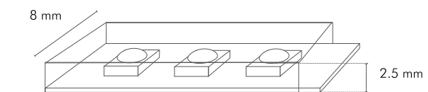
schéma en coupe de la bande
