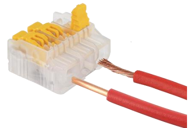
Insertion directe des fils rigides
