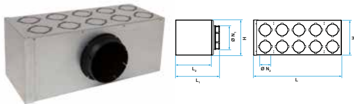
Caisson de répartition OPTIFLEX 20 piquages
