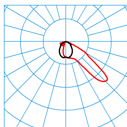
Jovie 50I-AM2L-LRA/6800-730 6G1 ET (CLO initial value) TX301425 ■ C0 - C180 ■ C90 - C270 DIN 5040: A40 UTE: 1,00 F CEN Flux Code: 47 91 100 100 100
