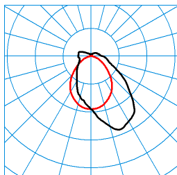
TugraHE 12 PAW 23-71/16ML-830 ET PC 23 (STAG13) TX425092 ■ C0 - C180 ■ C90 - C270 DIN 5040: B40 UTE: 0,86 E + 0,14 T CEN Flux Code: 48 77 92 86 100 13 32 64 14
