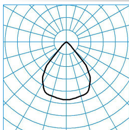
SNS RC5-HR1XFL-20-840 ■ C0 - C180
