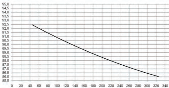
Courbe rendement
