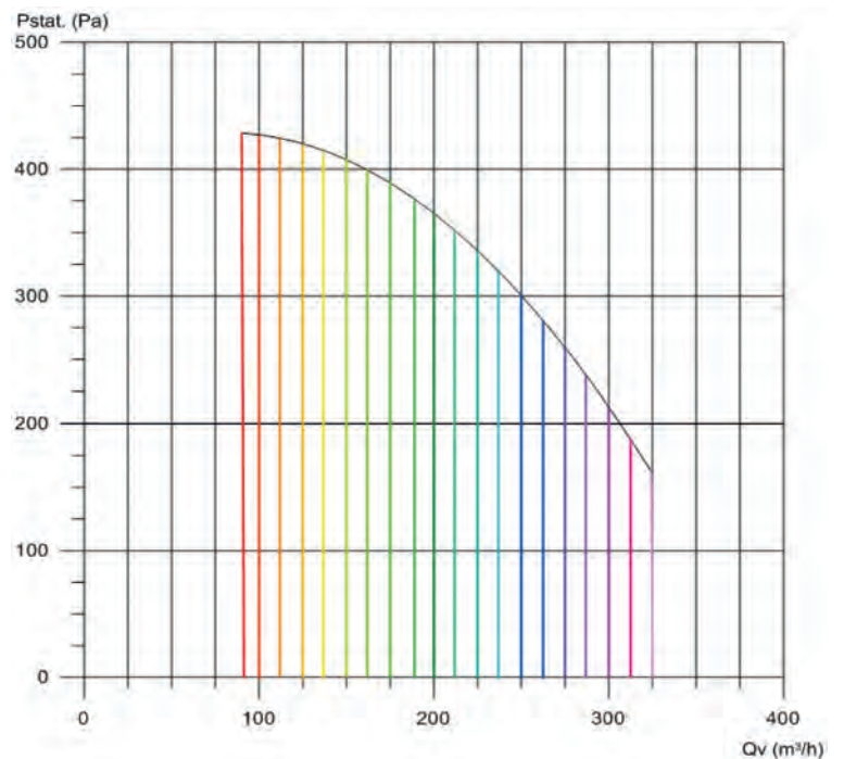
Courbe aéraulique
