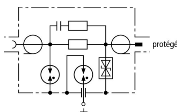
Schéma de principe du circuit UGKF BNC
