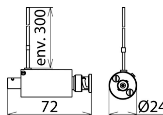
Dimensions UGKF BNC
