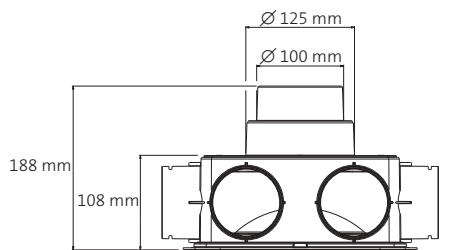
DB208 avec Multidiam Ø 100 - 125 mm
