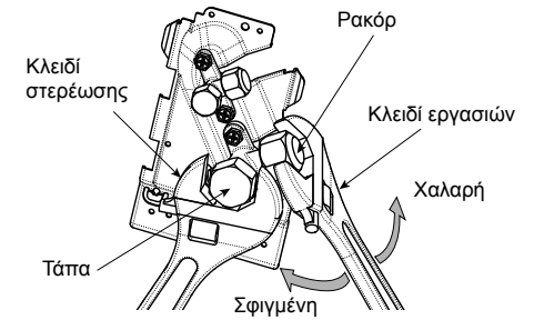
Βαλβίδα στην πλευρά αερίου
