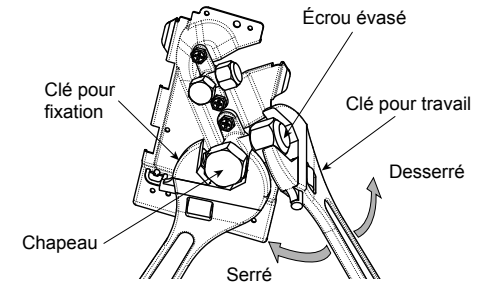
Soupape côté gaz
