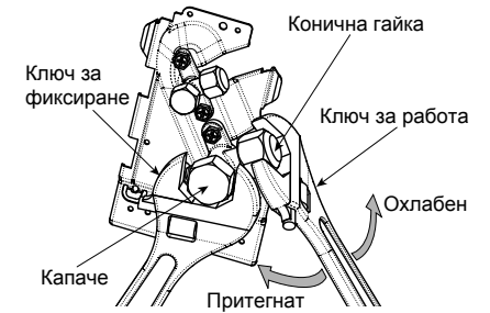
Клапан от газовата страна
