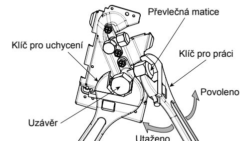
Ventil na straně plynu
