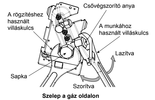
Szelep a gáz oldalon
