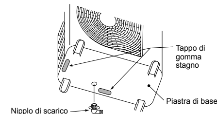
Tappo di gomma stagno (2 pezzi).
