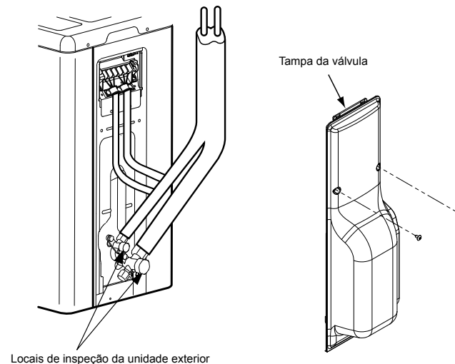
Locais de inspecção da unidade exterior
