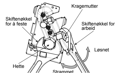
Ventil på gassiden
