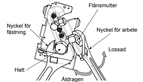
Ventil på gassidan
