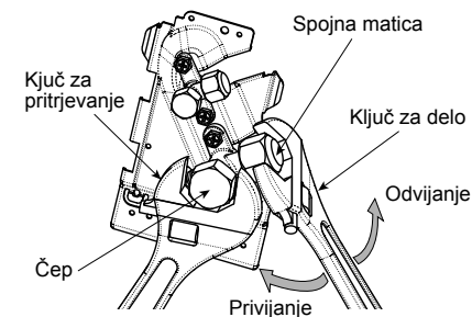
Ventil na plinski strani
