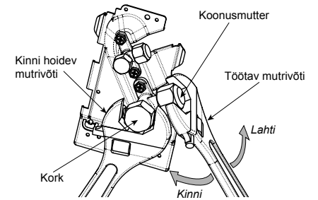
Ventiil gaasi poole
