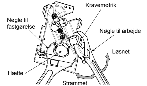
Ventil ved gasside
