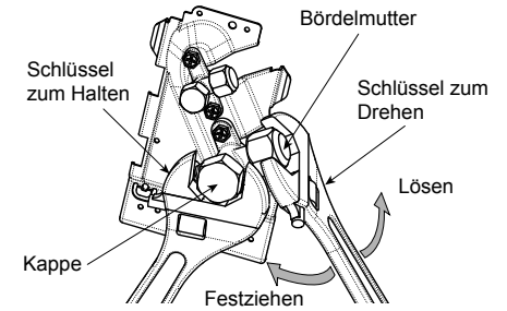
Ventil auf Gasseite
