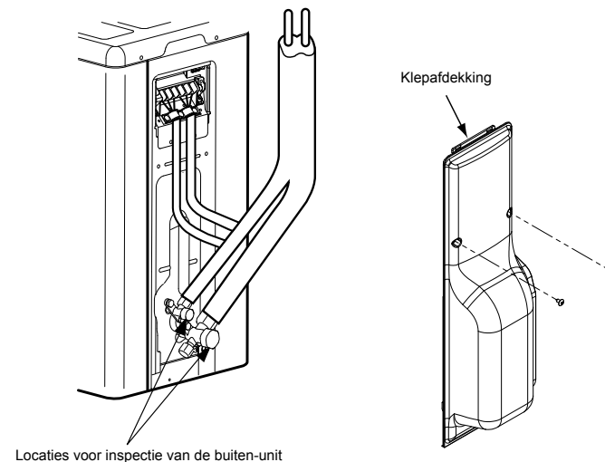
Locaties voor inspectie van de buiten-unit
