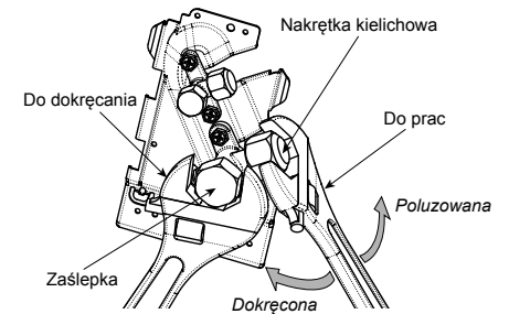
Zawór po stronie gazowej
