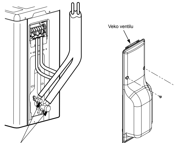
Miesto inšpekcie exteriérovej jednotky
