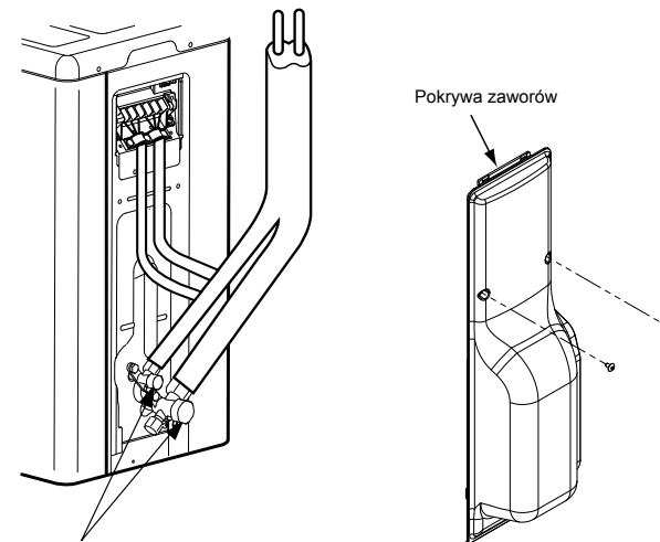
Lokalizacja inspekcji jednostki zewnętrznej
