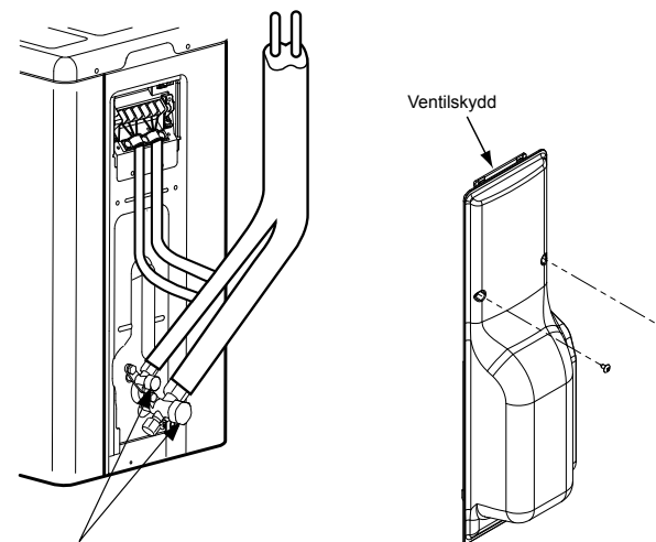
Inspektionsplatser för utomhusenhet
