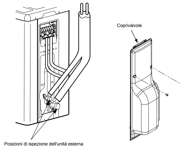
Posizioni di ispezione dell'unità esterna
