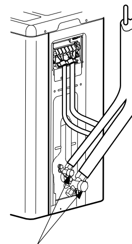
Inspektion af udendørsenhedens placering
