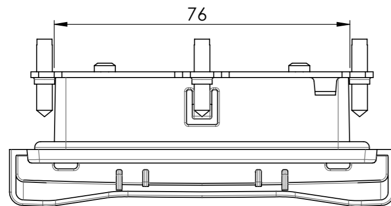
Oben / Top
