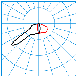
Jovie 70-FL1L-LR/6800-730 8G1 ET TX068653 ■ C0 - C180 ■ C90 - C270 DIN 5040: A40 UTE: 1,00 F CEN Flux Code: 38 80 98 100 100
