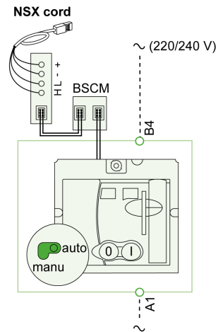
Avec commande électrique communicante (MTc)
