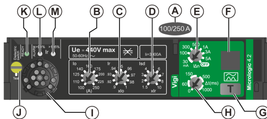
Version Déclenchement Micrologic 4.2 3P
