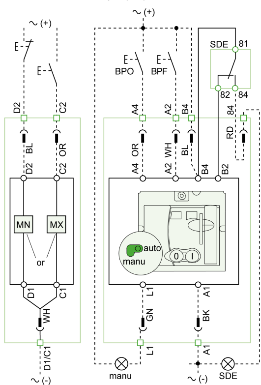
Avec commande électrique (MT)
