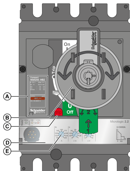
Porte d'armoire ouverte
