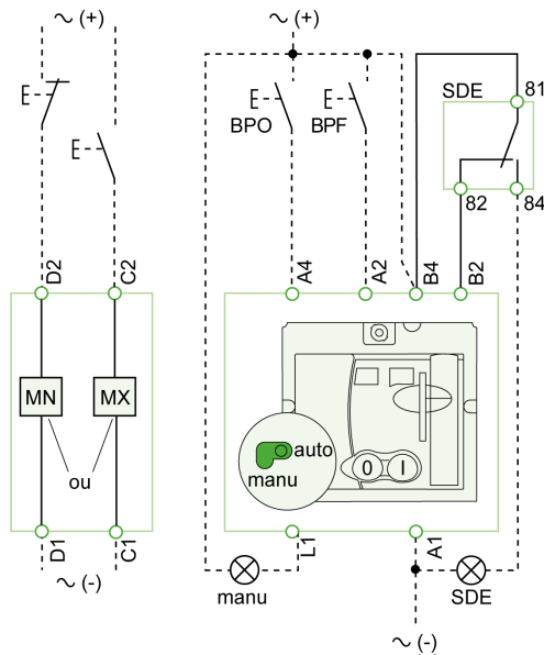
Avec commande électrique (MT)
