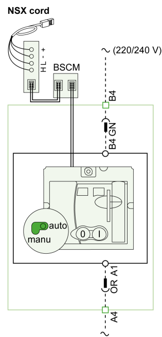
Avec commande électrique communicante (MTC)
