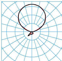
LuceoS S-U PAW-IL 300-830 03+LLWP(LEO2) TX245542 ■ C0 - C180 ■ C90 - C270 DIN 5040: E03 UTE: 0,08 D + 0,91 T CEN Flux Code: 53 86 96 8 100 49 82 98 92
