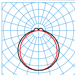
Olisq LWD2 DW 20-840 ETBLE +DMR IP54 IK TX430139
