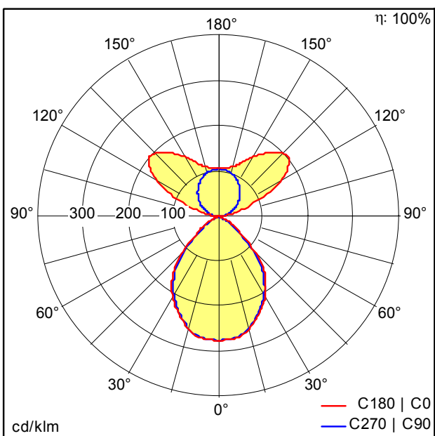
D43607AA_CLEVO_ID_LED_4400-830_L1280_LDO_SR_SRG.Idt
