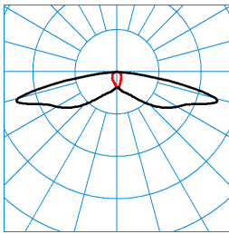
Jovie 50-SB3L-LR/1000-740 2G1 ET TX068581 ■ C0 - C180 ■ C90 - C270 DIN 5040: A20 UTE: 1,00 l CEN Flux Code: 29 61 91 100 100
