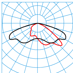
Jovie 70-AB7L-ML/5600-6800-730 8G1 ETDD (6800 lm) TX068719 ■ C0 - C180 ■ C90 - C270 DIN 5040: A30 UTE: 1,00 G CEN Flux Code: 34 71 96 100 100
