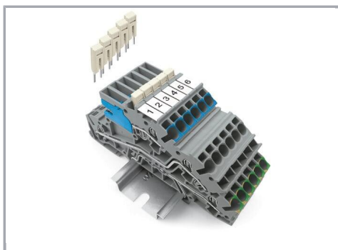
Contact de pontage horizontal pour pontage continu (2002-400)
