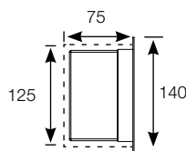
Dimensions d'encastrement : R x 125 mm x 75 mm
