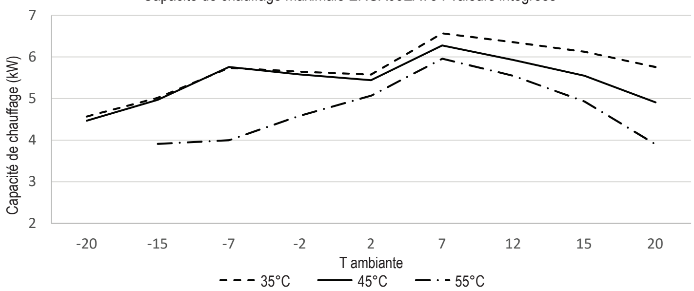
Capacité de chauffage maximale ERGA06EAV3 : Valeurs intégrées
