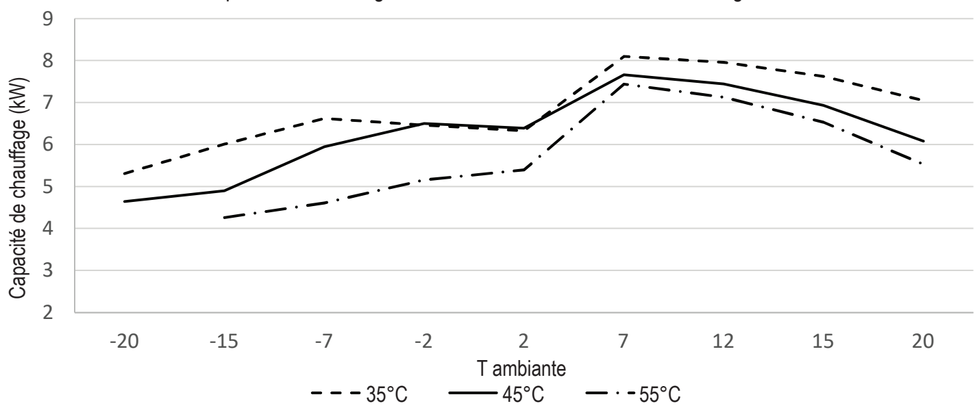
Capacité de chauffage maximale ERGA08EAV3 : Valeurs intégrées
