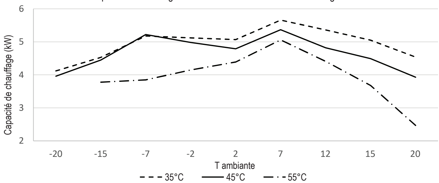
Capacité de chauffage maximale ERGA04EAV3 : Valeurs intégrées
