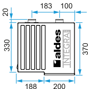
Encombrement C.Integra - Vue de dessus
