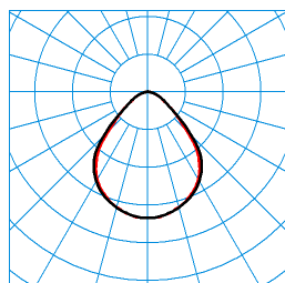
OpendoAct D2-L PW19 47-8 ETDD8 01 (ACTDCW) TX376849 ■ C0 - C180 ■ C90 - C270 UGR I = 18,4 UGR q = 18,7 DIN 5040: A50 UTE: 1,00 C CEN Flux Code: 65 90 98 99 100 14 43 71 1
