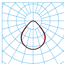
OpendoAct D2-L PW19 47-8 ETDD8 01 (ACTDSU) TX377065 ■ C0 - C180 ■ C90 - C270 UGR I = 18,4 UGR q = 18,7 DIN 5040: A50 UTE: 1,00 C CEN Flux Code: 65 90 98 99 100 14 43 71 1
