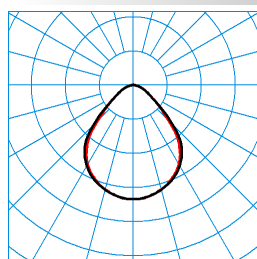
OpendoAct D2-L PW19 47-8 ETDD8 01 (ACTDWW) TX377665 ■ C0 - C180 ■ C90 - C270 UGR I = 18,4 UGR q = 18,7 DIN 5040: A50 UTE: 1,00 C CEN Flux Code: 65 90 98 99 100 14 43 71 1
