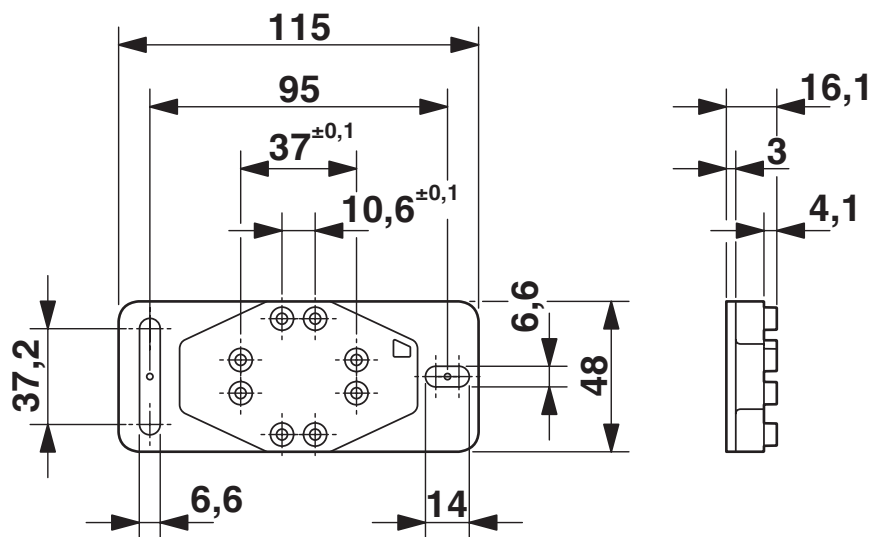
Dessin coté
