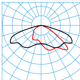
Jovie 70-AB7L-LRA/24000-740 24G1 ET TX068639 ■ C0 - C180 ■ C90 - C270 DIN 5040: A30 UTE: 1,00 G CEN Flux Code: 35 73 97 100 100
