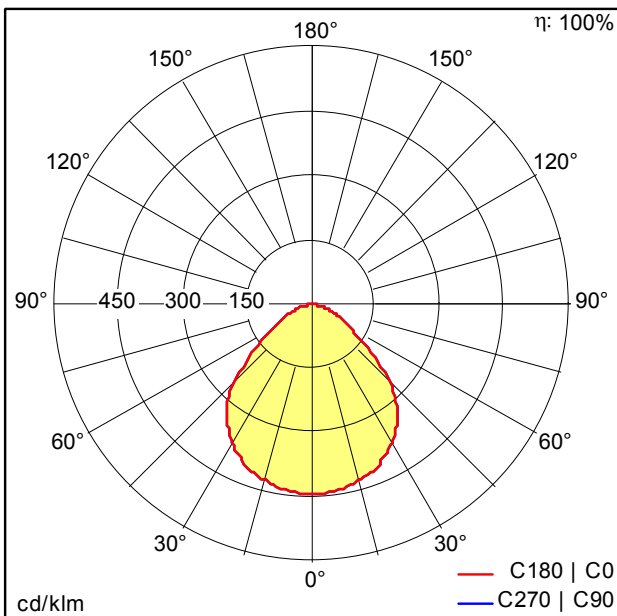
D37457AA_u_ONDA2_E_LRO_D1150_LED16000-830.idt
