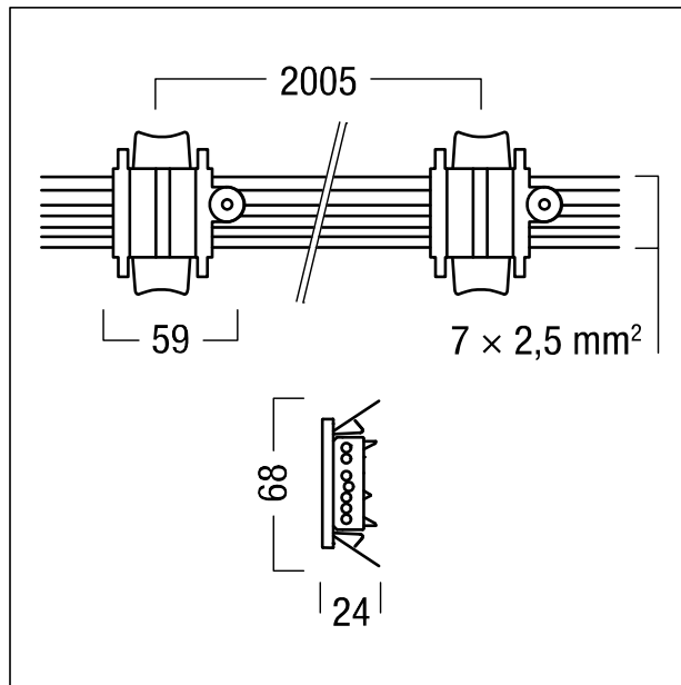
ZS_TRS_M_Verdrahtung_7pol_2000.wmf
