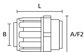
Raccord FlexiGuard, droit avec filetage tournant
