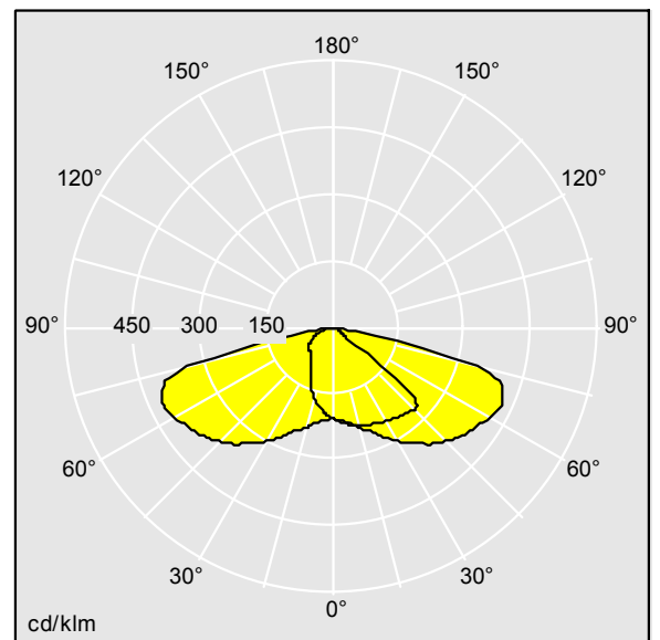
TL_IS36L70NR730.idt
