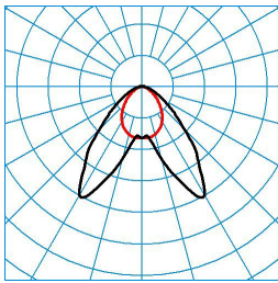
ELINE FL LDAW100 840 L225 1 20
