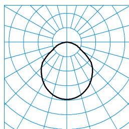
Inplana C07 OTA25 2000-840 01 + C07 ZPF - T WR TX049217 ■ C0 - C180 UGR I = 24,3 UGR q = 24,3 DIN 5040: A40 UTE: 1,00 D CEN Flux Code: 52 83 96 100 100 0 0 0 0
