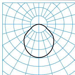
Inplana C07 OTA25 2000-840 01 TX372302 ■ C0 - C180 UGR I = 24,3 UGR q = 24,3 DIN 5040: A40 UTE: 1,00 D CEN Flux Code: 52 83 96 100 100 0 0 0 0
