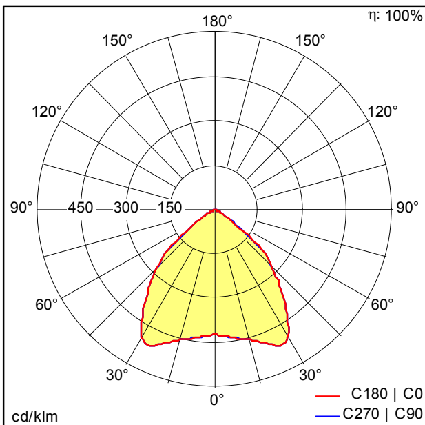
D43022_MIRL_NIV_3800-840_M600Q_WB_LDO_WH.Idt
