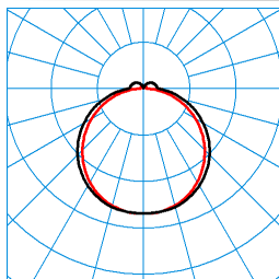
LightP G2 3P OTR 8000-830 03 NO TX056241
