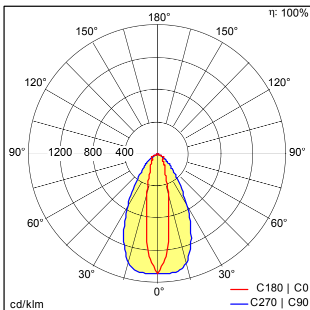
D44423AA_TEC_LED8000-840_L1000_NB_LDE_SR_IP.idt
