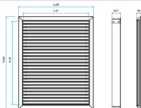
Grille de reprise T.One® AquaAIR/T.One® AIR
