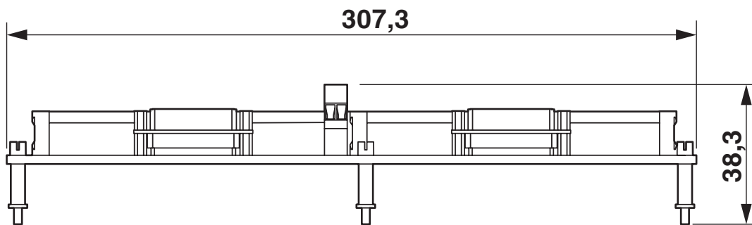
Dessin coté
